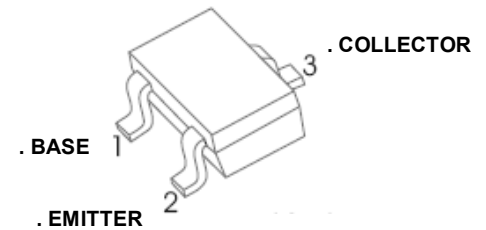
SOT - 323
